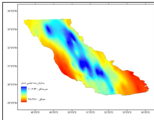
و-مدل سازی بارش با استفاده از کریجینگ عام
