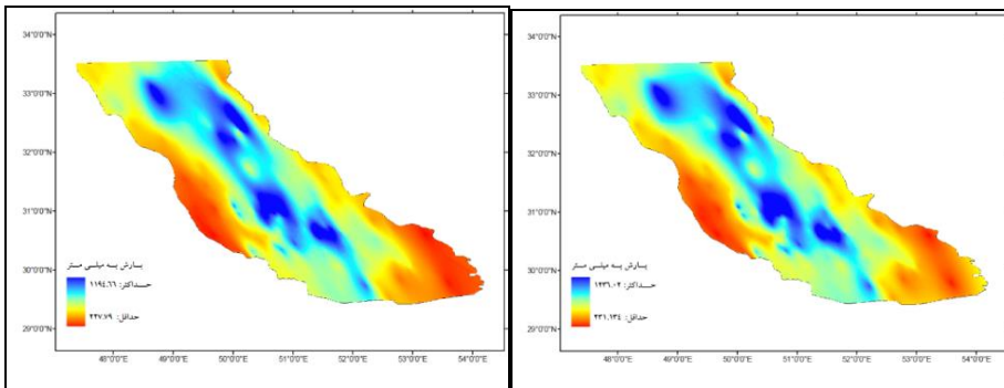
ج-مدل سازی بارش با استفاده از کریجینگ ساده د-مدل سازی بارش با استفاده از کریجینگ معمولی
