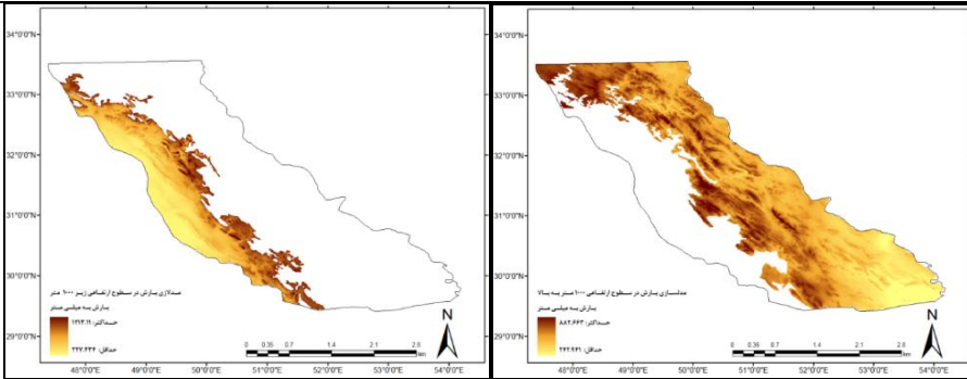
الف-مدل سازی بارش در سطوح ارتفاعی ۰ تا ۱۰۰۰ متر ب-مدل سازی بارش در سطوح ارتفاعی ۱۰۰۰ متر به بالا
